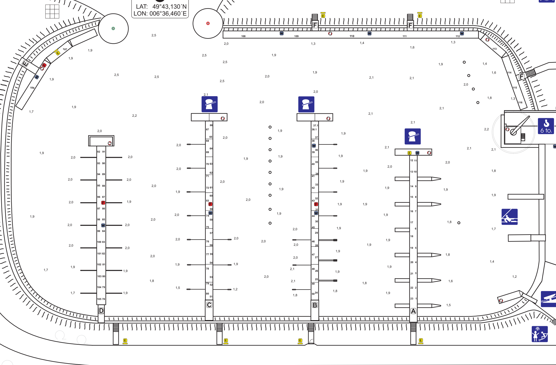
Vermessungsplan Yachthafen Trier- Monaise, Wassertiefe bei Normalstand, Planungsstand: 08.11.2018
